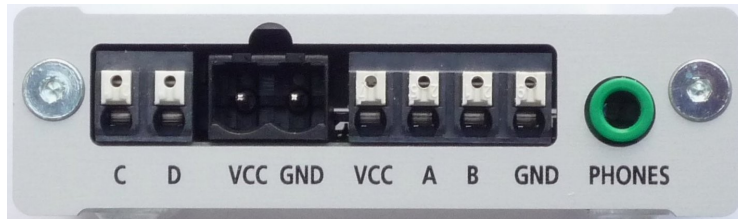
Rückansicht des MM-2214
